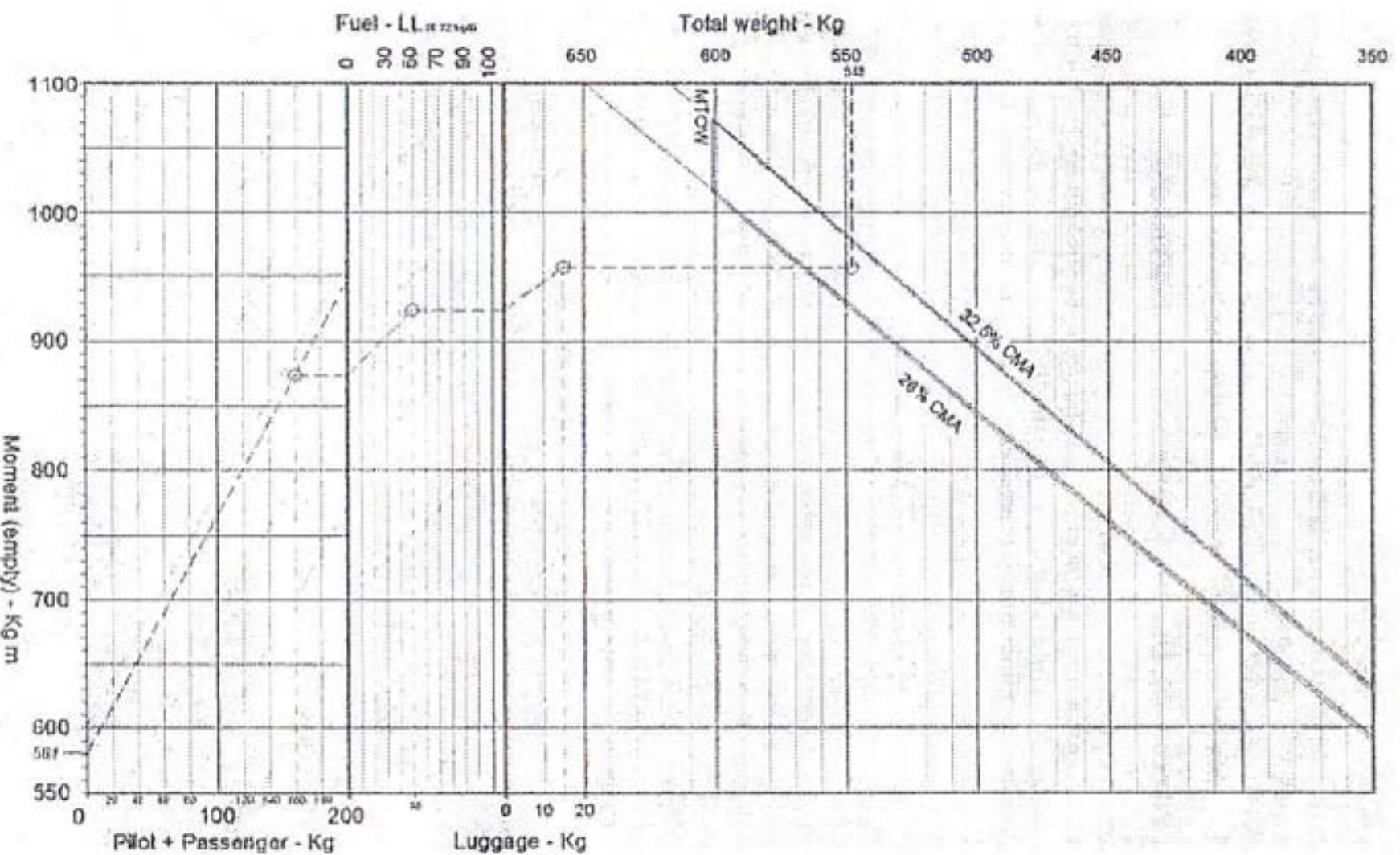
fig. 6-2 Tableau masse & centrage
